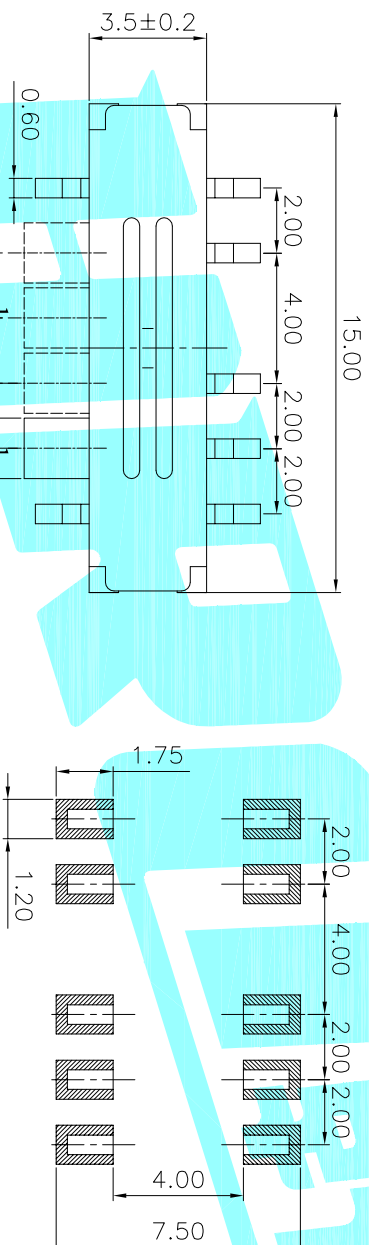
P.C.B layout
