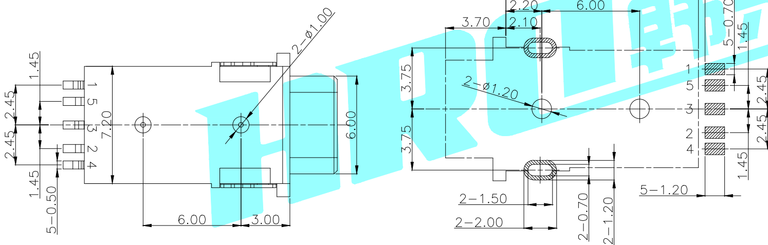
P.C.B. Layout
